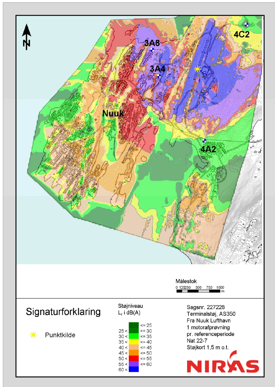
Figur 5.35: Terminalstøj, motorafprøvning Helikopter, nat. Punkterne 3A 4, 3A8, 4A2 er boligområder. Område 4C2 er område ud- lagt til anstaltområde. Støj- grænsen på 35 dB(A) over- holdes kun ved boliger i de grønne områder og er således overskredet ved områderne 3A8 og 3 A4 samt ved Anstal- ten (4C2)
