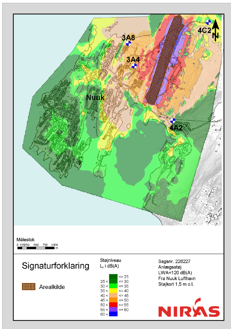
Figur 5.27: Støjbidrag fra anlægsarbejder (worst case, fuld aktivitet).
