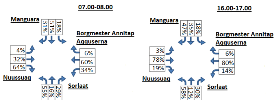
Figur 5.16: Krydstælling i rundkørslen Manguara/Nuussuaq/Sor- laat/Borgmester Annitap Aqq. foretaget i 2013. Der er angivet morgen- og eftermiddags- spidstimen.
