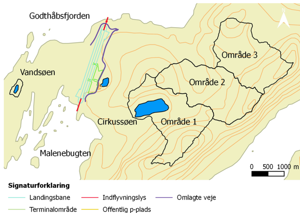
Figur 5.45: Oversigtskort, der viser den planlagte placering af lufthavnen og vandspærrezone om Qallusuaq (Cirkussøen), der forsyner Nuuk med drikkevand.
