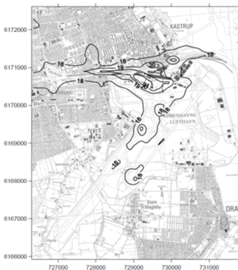
Figur 5.44: Overordnet geografisk fordeling af årsmiddelværdien af PM_{2,5} ( \mu g/m^3 ). Spredningsberegninger med OML i gitternet på 150 m.
