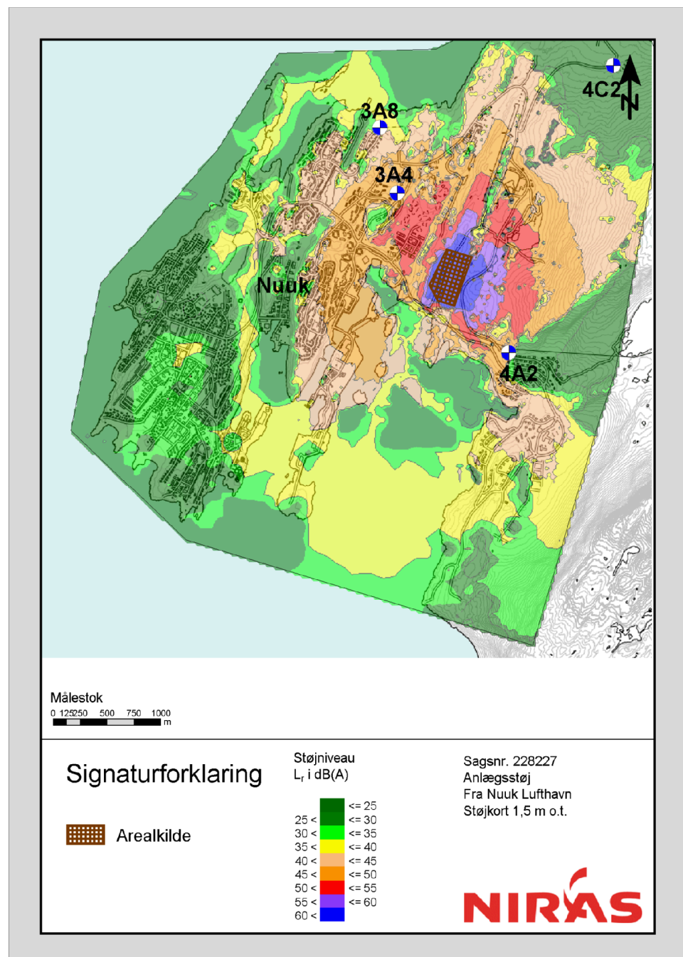
Figur 1.3: Støjbidrag fra anlægsarbejder (worst case, fuld aktivitet i det sydlige område).
