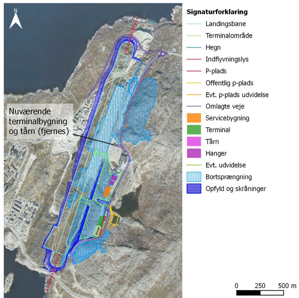
Figur 3.5: Udvidelse af Nuuk Lufthavn med landingsbane, terminal- område inkl. byggefelter for service bygning, terminal og tårn. Derudover er områder for bortsprængning af fjeld samt opfyldt med sprængsten vist.
