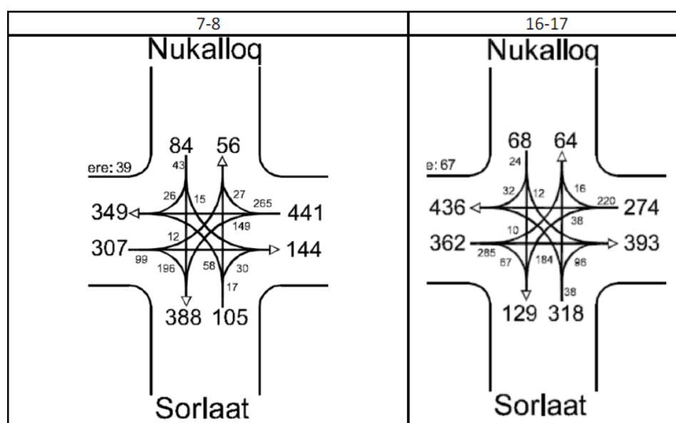
Figur 5.10: Krydstælling i rundkørslen Borgmester Anniitap Aqquserna/ Sorlaat/ Manguaraq/Nuussuaq foreta- get i 2013. Der er angivet morgen- og eftermiddags- spidstimen. (Via Trafik, 2013).
