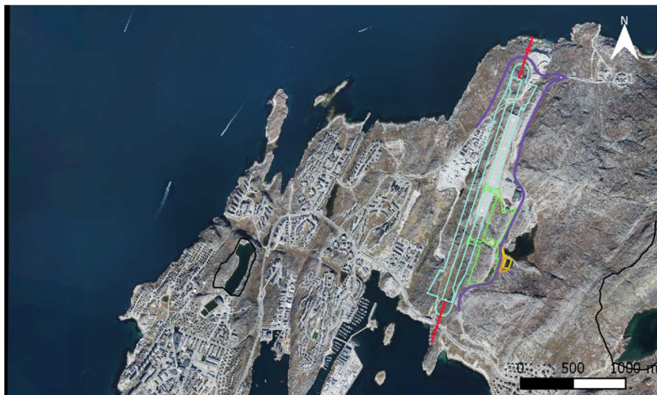
Figur 3.4: Oversigt over udvidelsen af Nuuk Lufthavn med landings- bane, terminalområde, lan- dingslys m.m. samt offentlig P-plads og omlagte veje.
