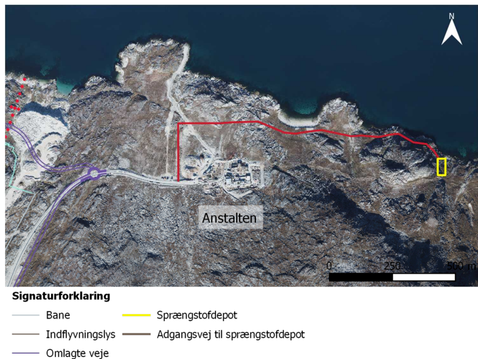
Figur 3.10: Planlagt beliggenhed af nyt sprængstofdepot til brug i forbindelse med anlægsfasen.
