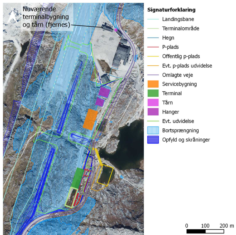
Figur 3.6: Oversigt over terminalområdet med byggeplaner for servicebygning, terminal, tårn. Derudover er nuværende terminalbygning og tårn fremhævet (disse fjernes).
