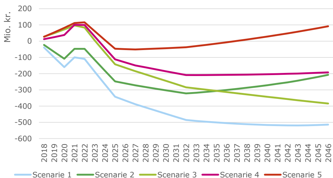
Figur 9: Akkumuleret driftsbudget for de fem scenarier baseret på årlige anlægsomkostninger, driftsomkostninger samt driftsindtægter.
