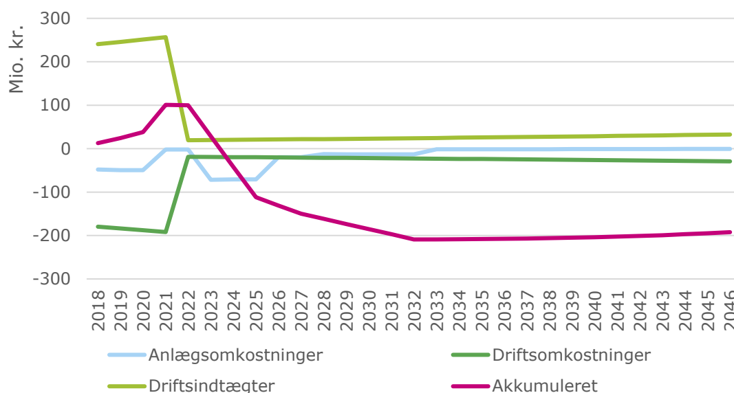
Figur 7: Anlægsomkostninger, driftsomkostninger, driftsindtægter samt akkumuleret driftsresultat for scenarie 4
